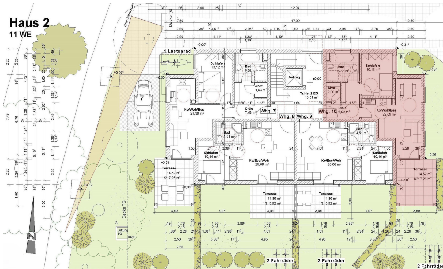
BI-25-05-W10-Plan Erdgeschoss
