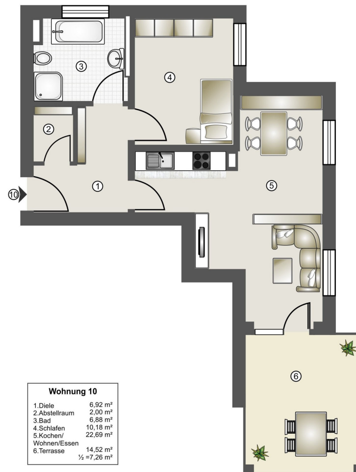
BI-25-05-W10-Grundriss
