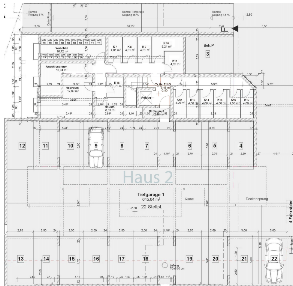
BI-25-05-W11-Tiefgaragenplan
