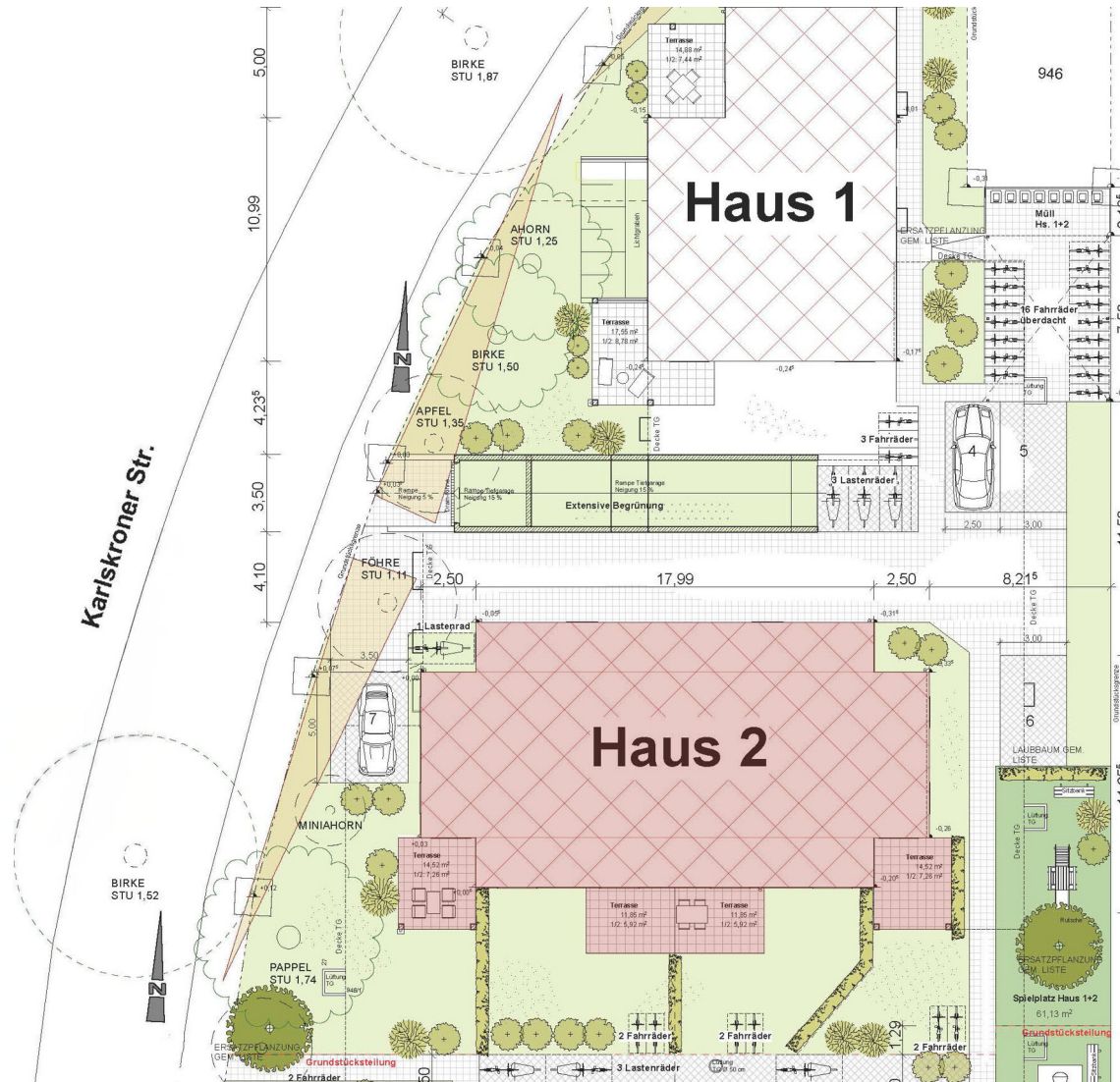
BI-25-05-W11-Lageplan_H1-2
