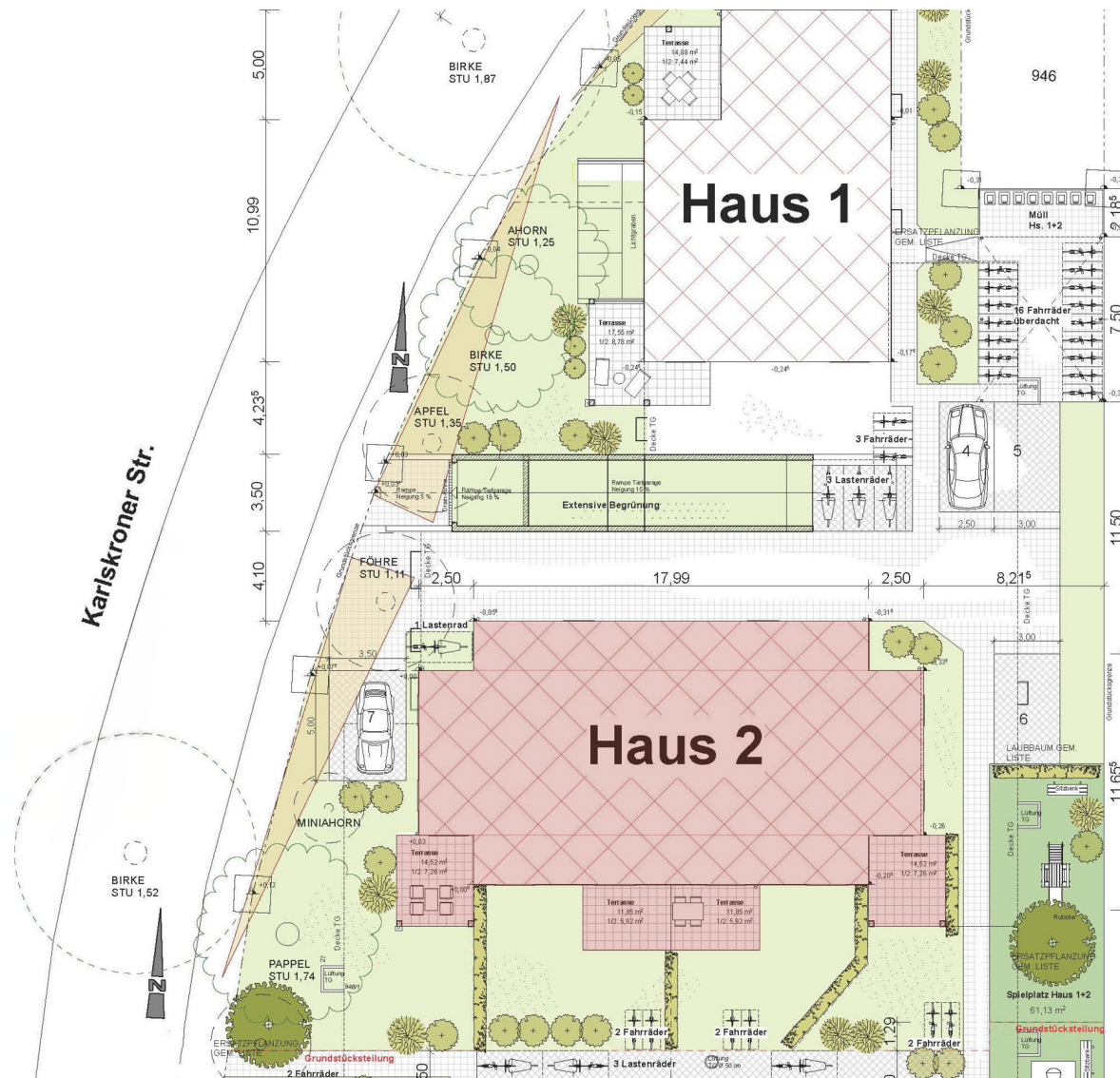
BI-25-05-W12-Lageplan_H1-2
