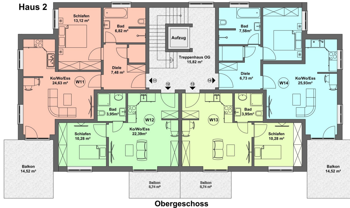
BI-25-05-KK 27a_H2_W11-14_OG_Grundriss
