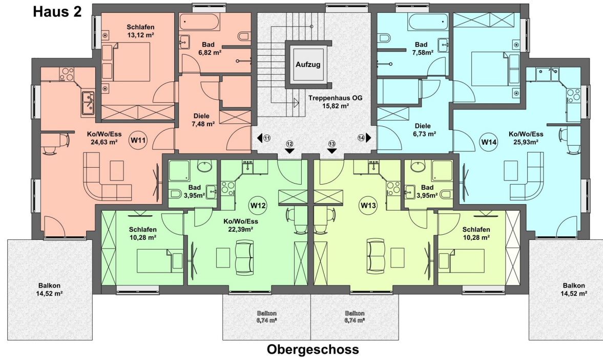
BI-25-05-KK 27a_H2_W11-14_OG_Grundriss
