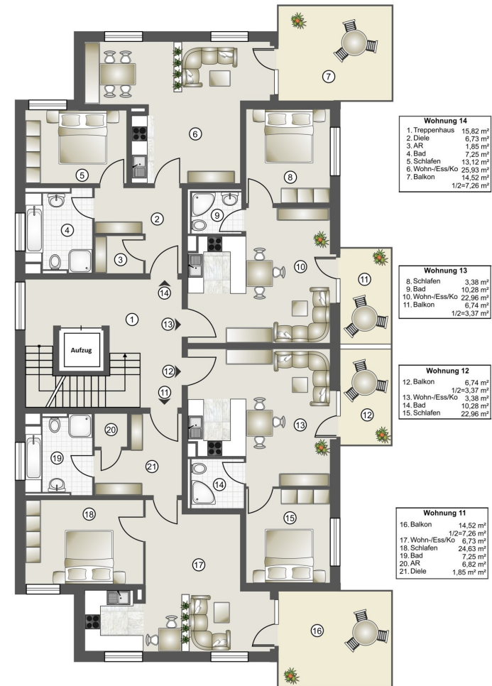
BI-25-05-W14-Geschossgrundriss
