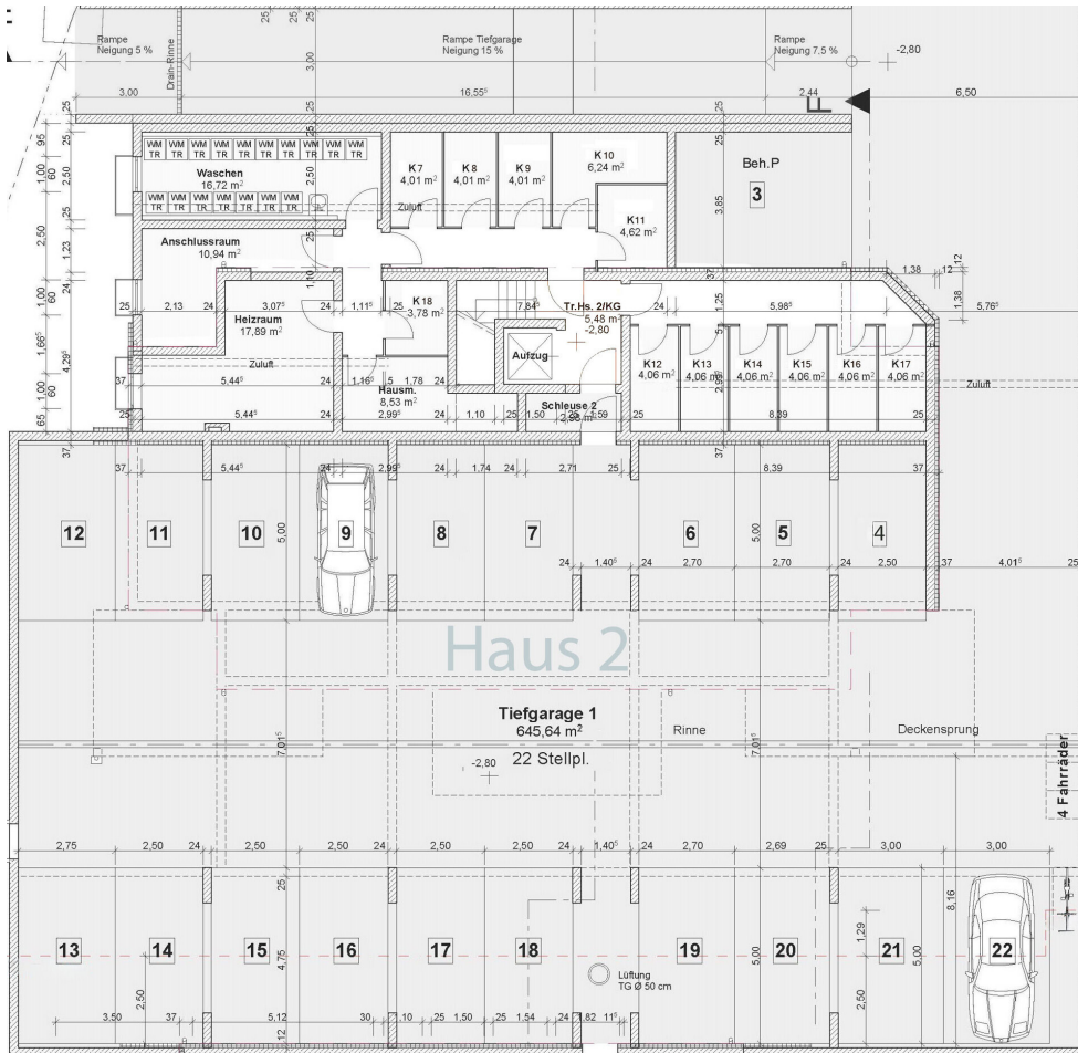
pic13_BI-25-05-W7-Tiefgaragenplan
