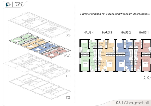
Grundriss Obergeschoß
